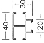
Dobbeltstyr
